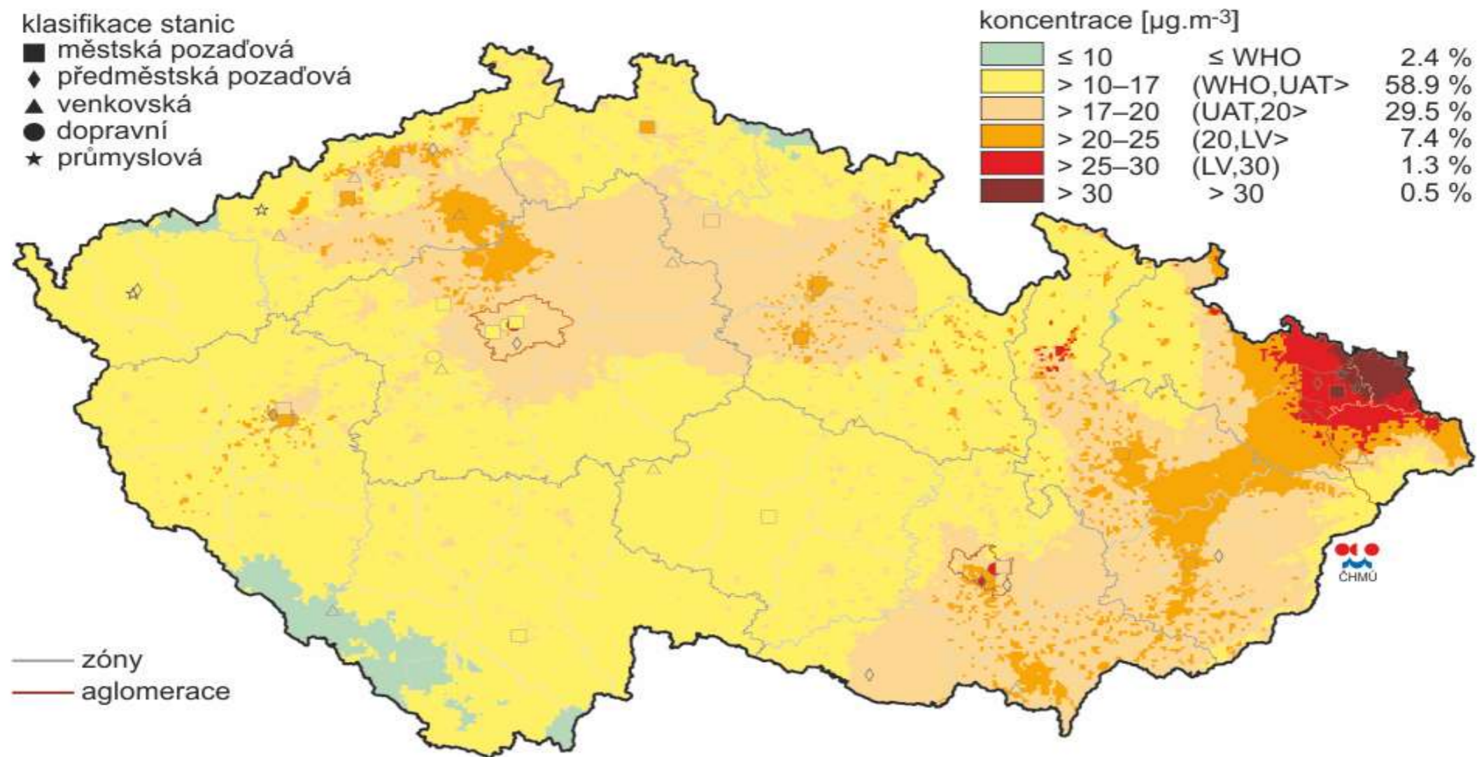
Obr. IV.1.4 Pole roční průměrné koncentrace PM 2,5 , 2014
