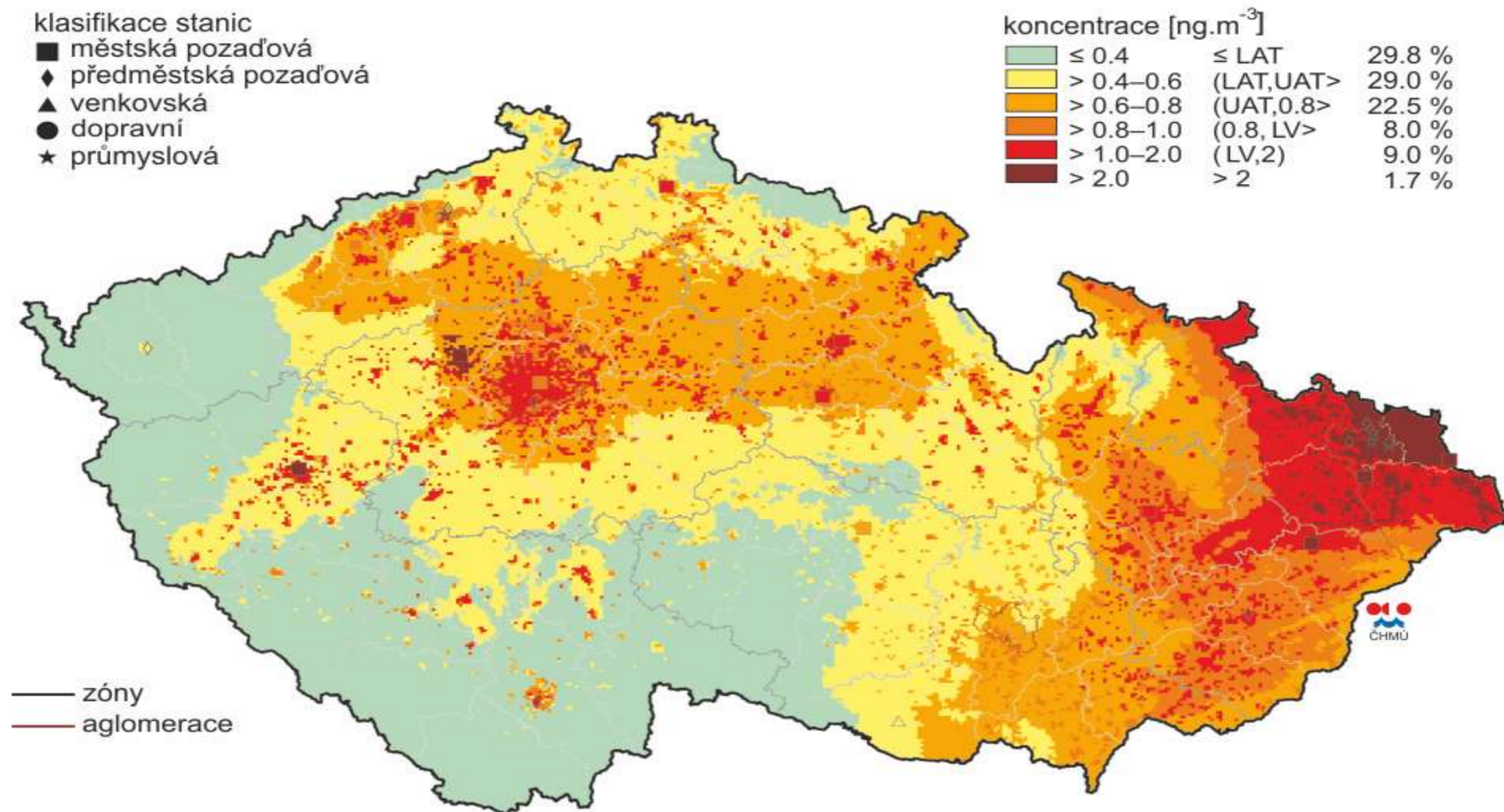
Obr. IV.2.1 Pole roční průměrné koncentrace benzo[a]pyrenu, 2014
