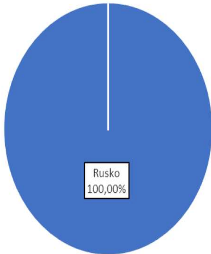
Dovoz podle zemí - zemní plyn, 2020
