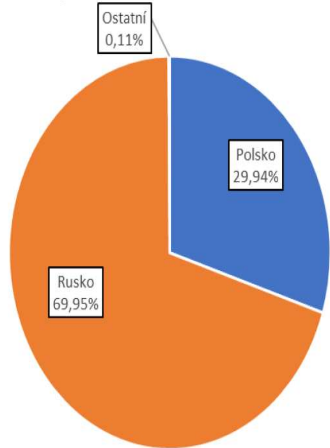
Dovoz podle zemí - antracit, 2020
