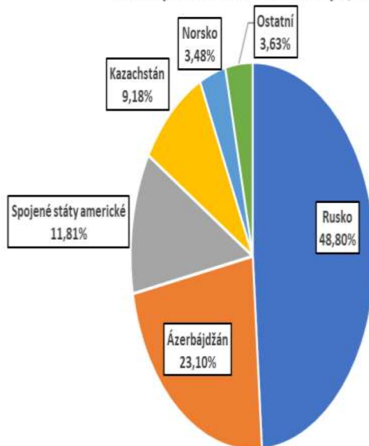
Dovoz podle zemí - surová ropa, 2020
