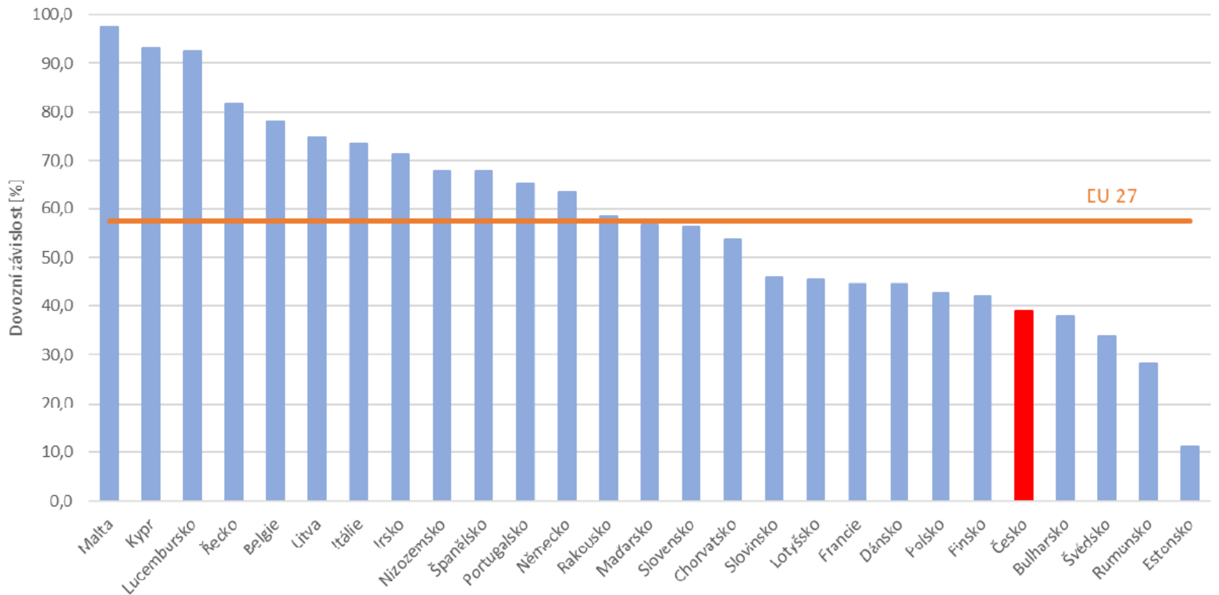
Energetická dovozní závislost zemí EU 27, 2020
