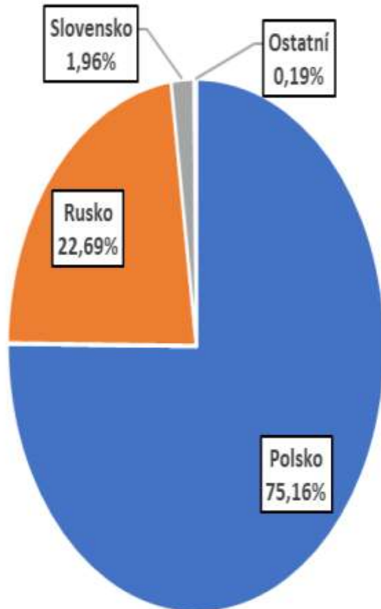
Dovoz podle zemí - černé uhlí energetické, 2020
