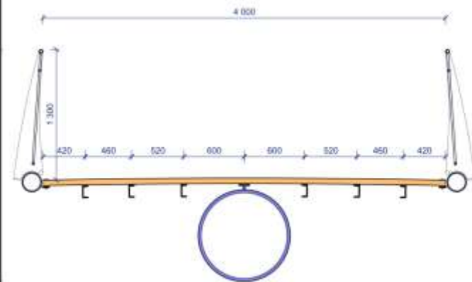
Příčný řez v poli
