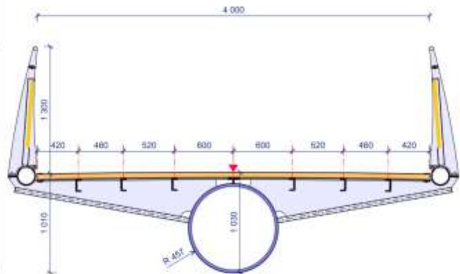
Příčný řez nad podpěrou
